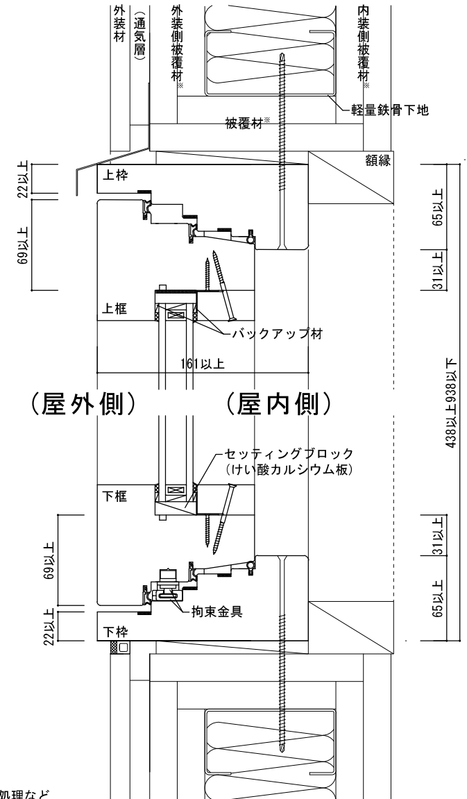
図9-8 鉛直断面図
