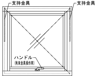
図9-6 屋内側姿図
