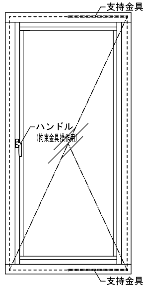
図8-10 屋内側姿図
