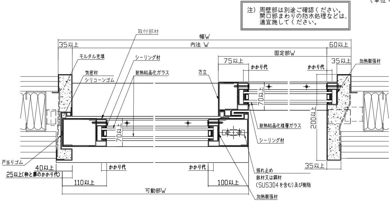
図 2-③ 水平断面図
