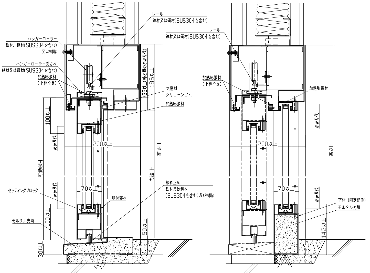
図 2-④ 鉛直断面図 (可動部側 (閉鎖時))
