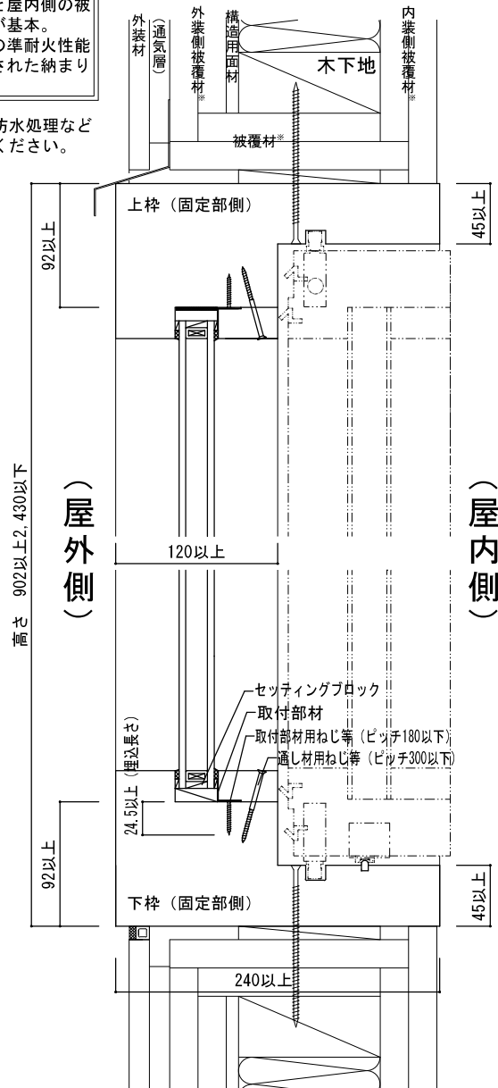
図10-⑦ 鉛直断面図〔固定部側(開放時)〕
