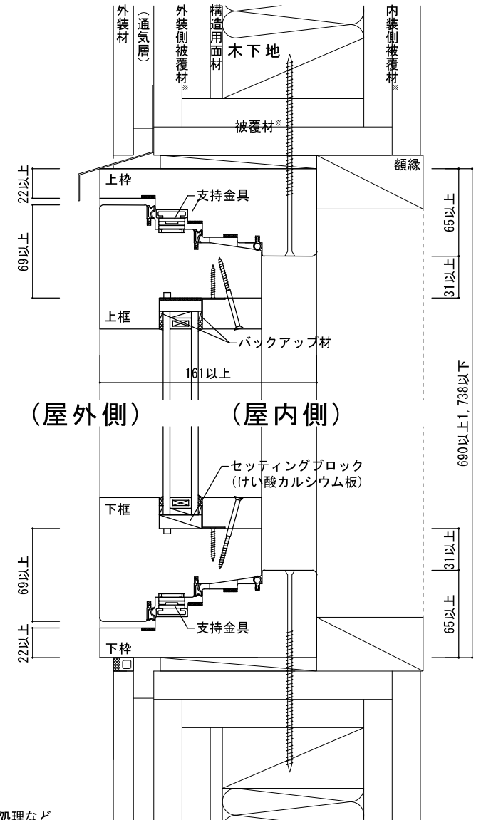
図 8 - ④ 鉛直断面図
