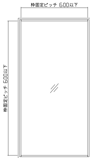
図 1-① 姿図
