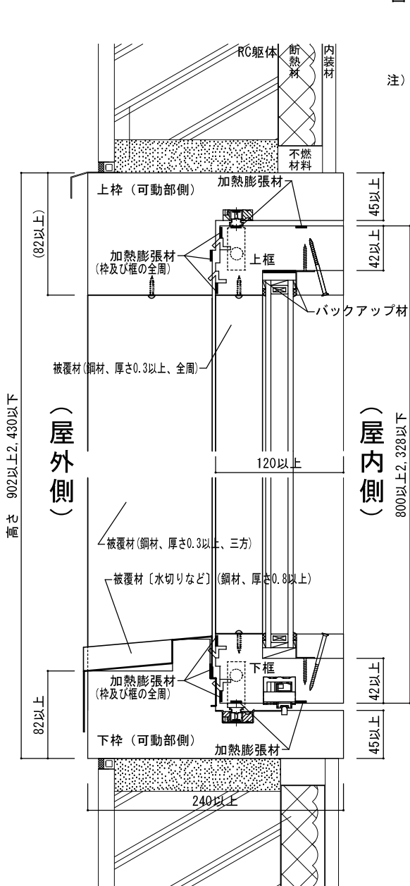
図10-⑫ 鉛直断面図〔可動部側（閉鎖時）〕
