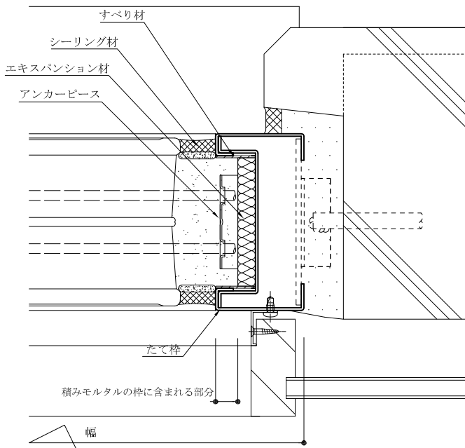
図5-⑤ 水平断面図
