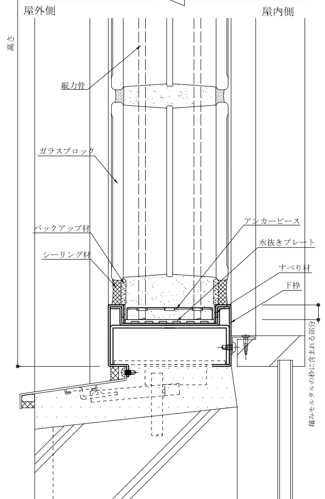
図5-⑥ 鉛直断面図
