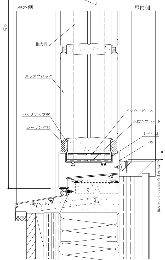
図6-③ 鉛直断面図
