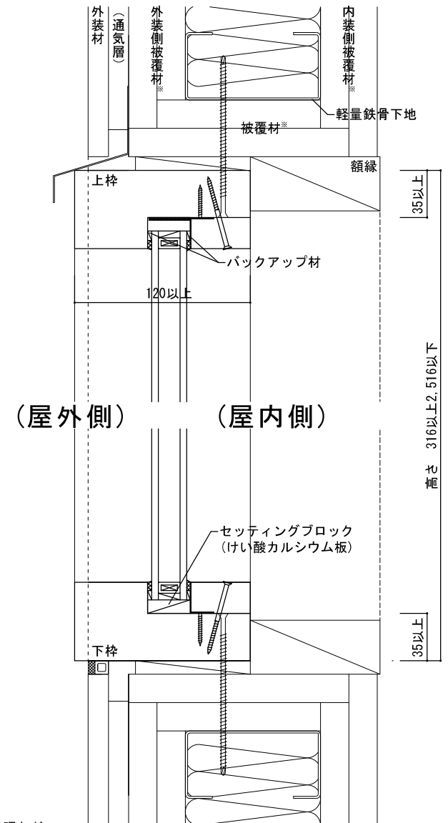
図 7-8 水平断面図
