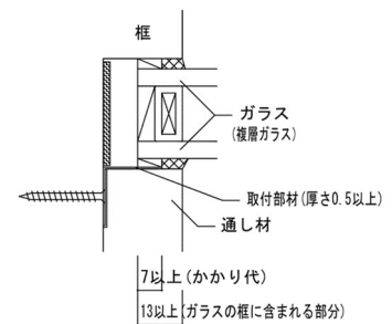
ガラスまわり寸法説明図
