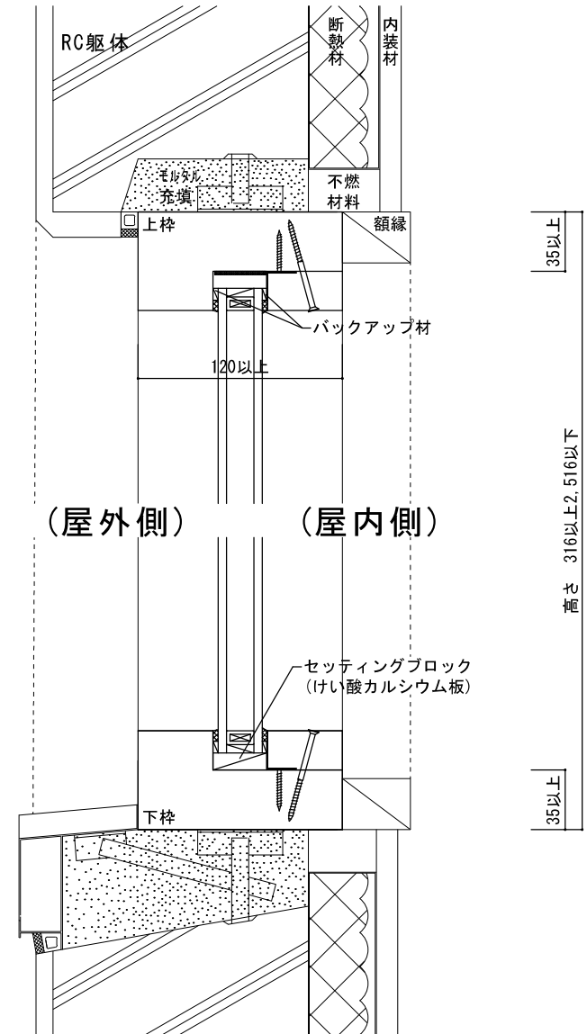
図 7-12 水平断面図
