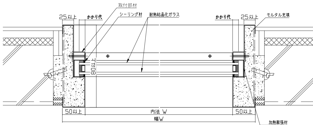
図 1-5 水平断面図
