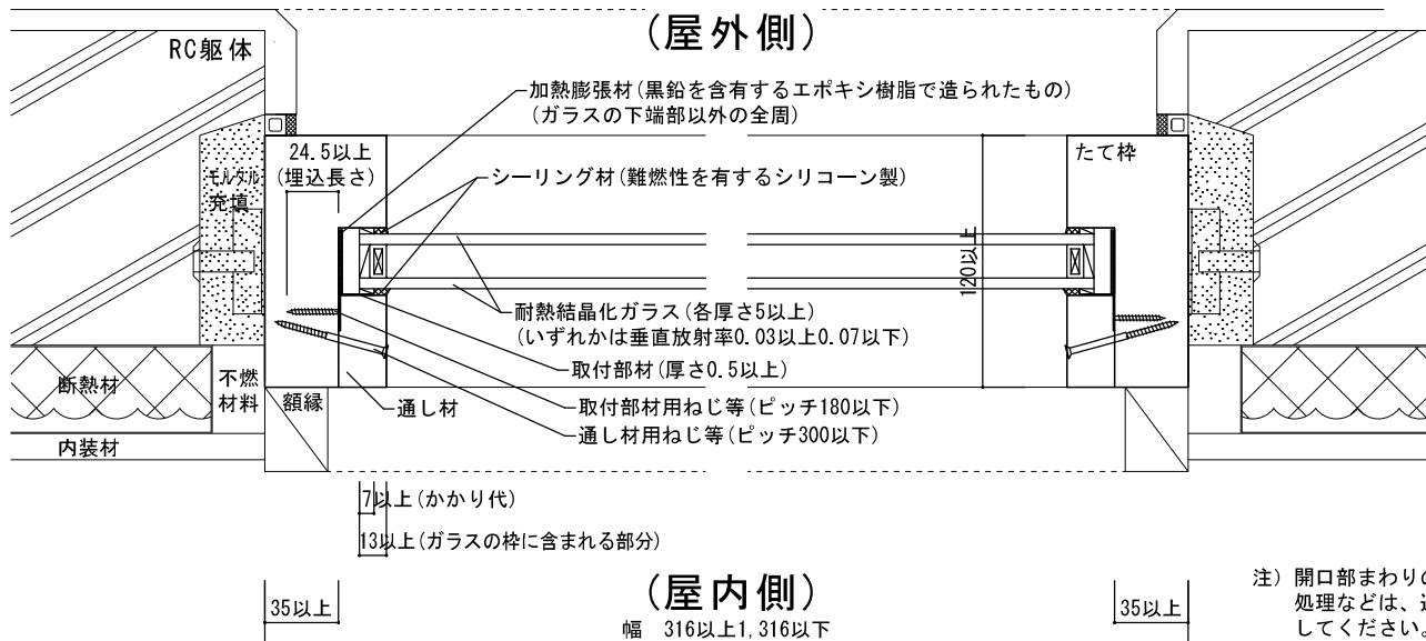
図 7-11 水平断面図
