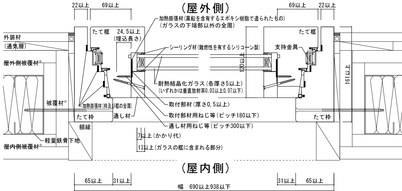
図9-7 水平断面図
