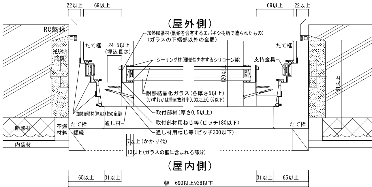
図9-11 水平断面図
