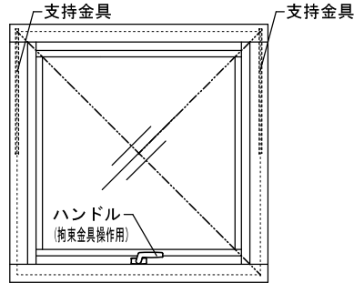
図9-10 屋内側姿図
