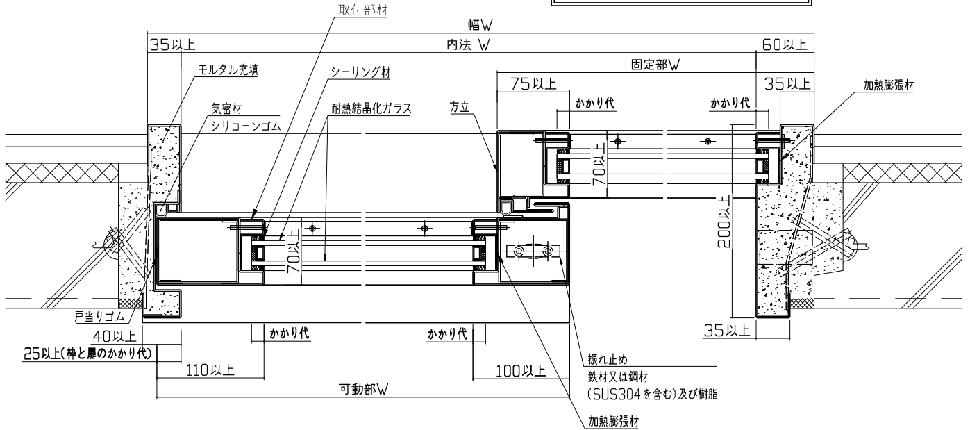
図 2-⑥ 水平断面図
