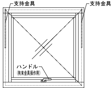
図9-② 屋内側姿図
