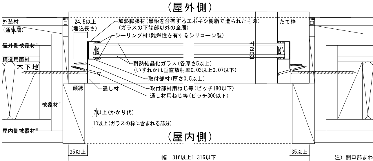
図 7-3 水平断面図
