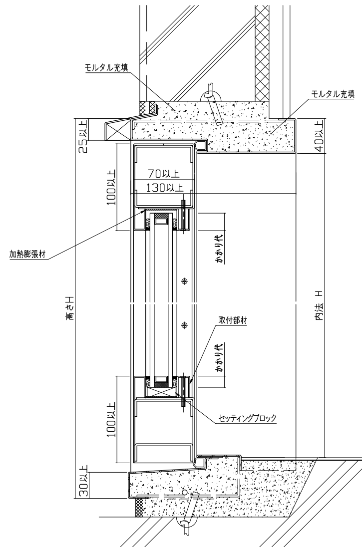
図 3-6 鉛直断面図
