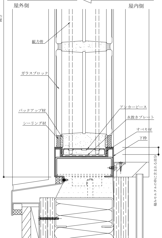
図5-③ 鉛直断面図
