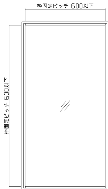
図 1-4 姿図
