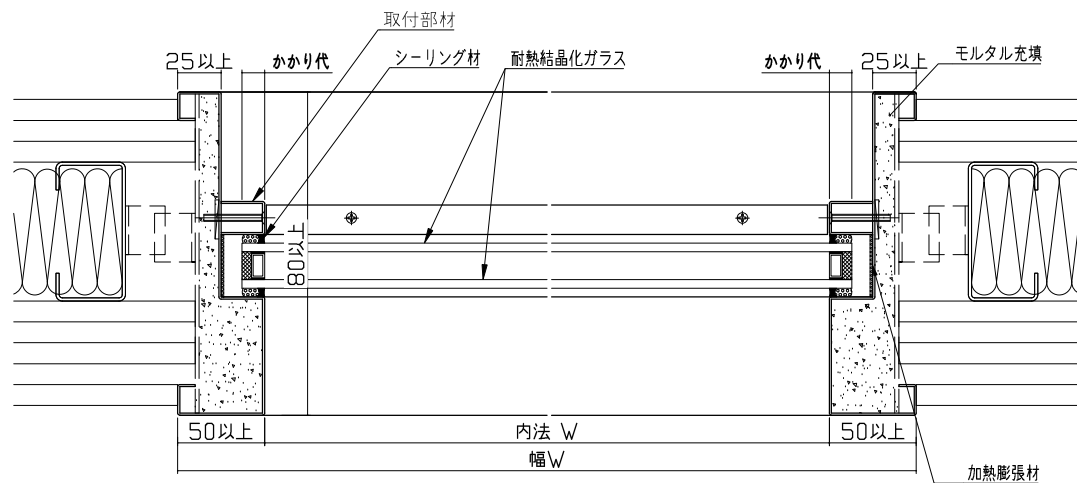
図 1-② 水平断面図
