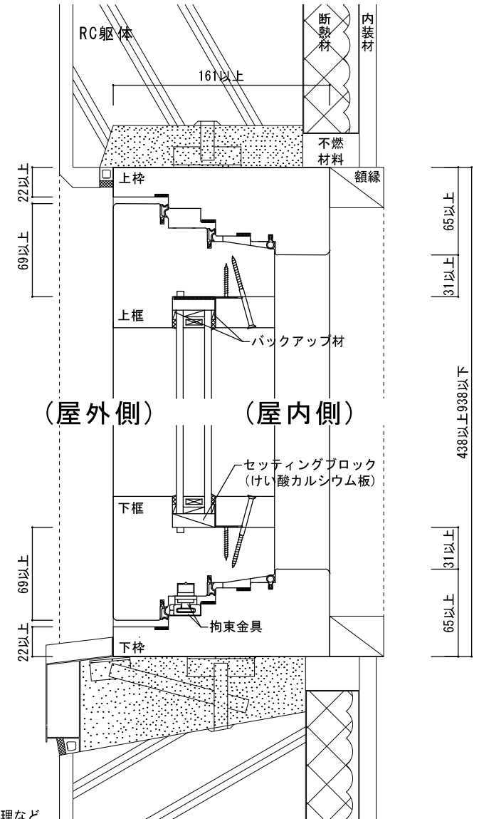
図9-12 鉛直断面図
