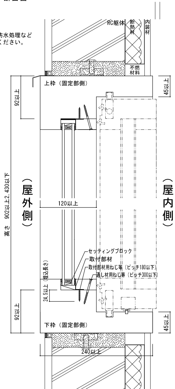
図10-⑬ 鉛直断面図〔固定部側（開放時）〕
