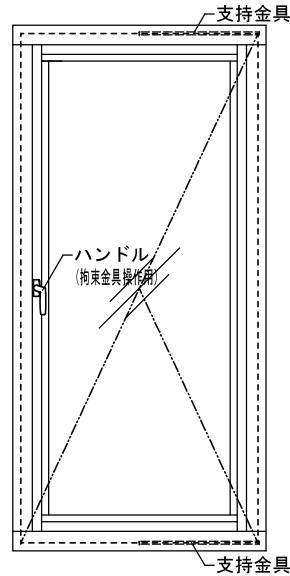
図 8 - ⑥ 屋内側姿図
