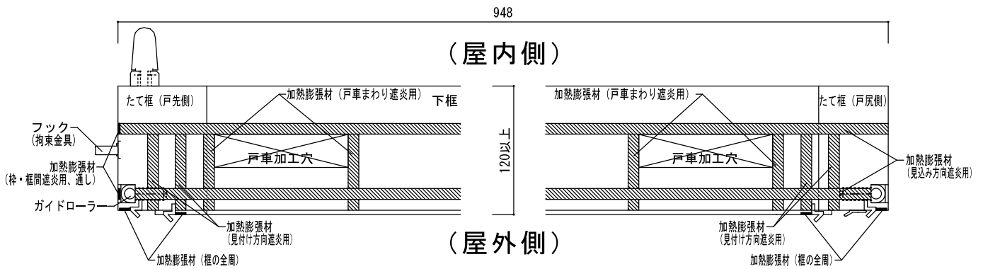
図10-④ 可動部、下面図
