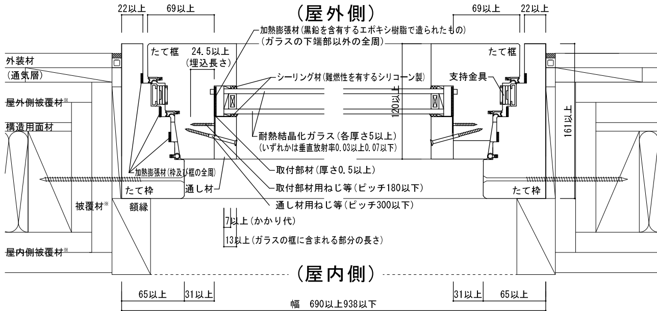
図9-③ 水平断面図
