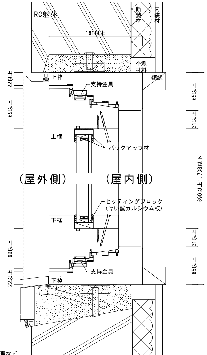
図8-12 鉛直断面図
