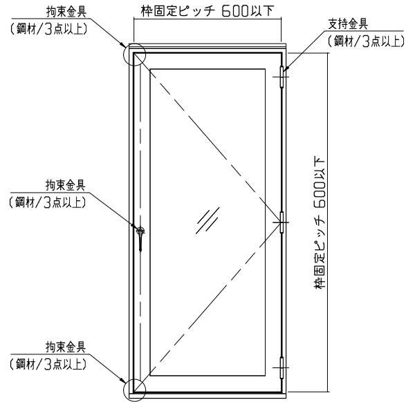
図 3-1 姿図
