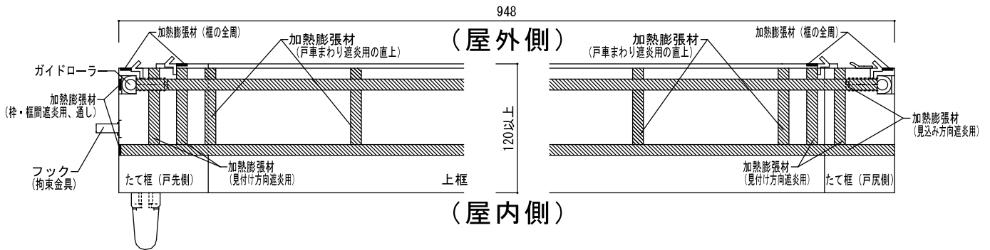
図10-③ 可動部、上面図
