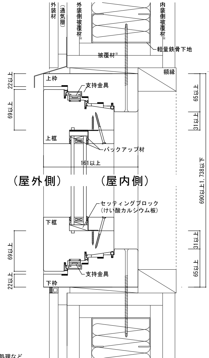
図 8 - ⑧ 鉛直断面図
