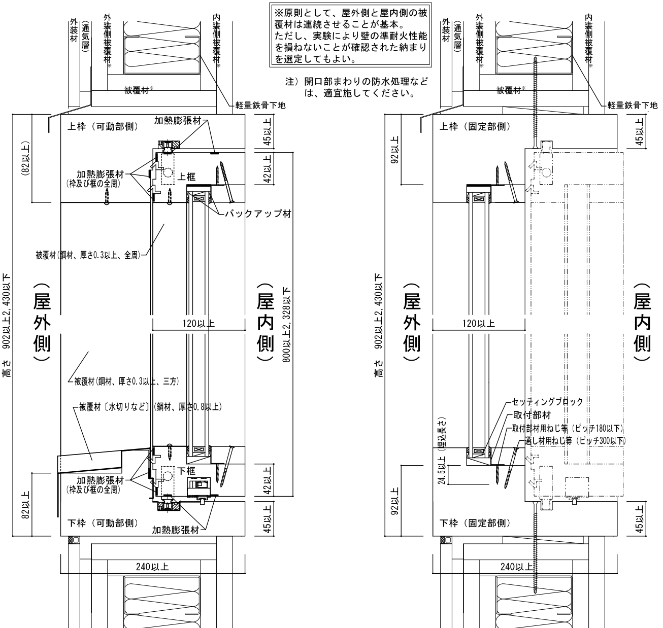
図10-⑨ 鉛直断面図〔可動部側(閉鎖時)〕
