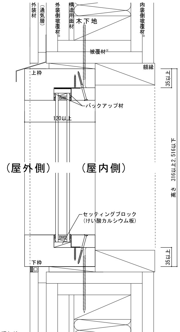
図 7-4 水平断面図
