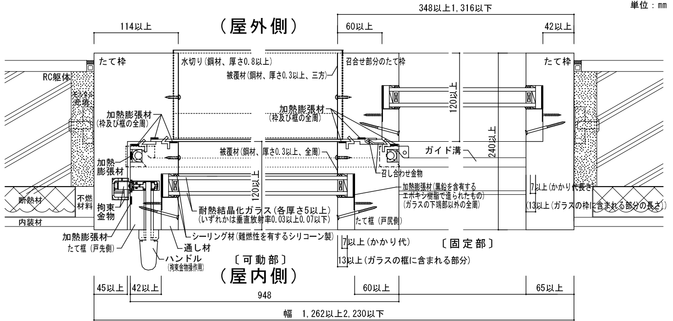
図10-⑪ 水平断面図
