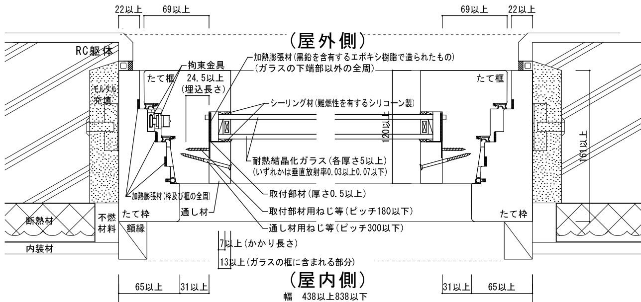
図8-11 水平断面図
