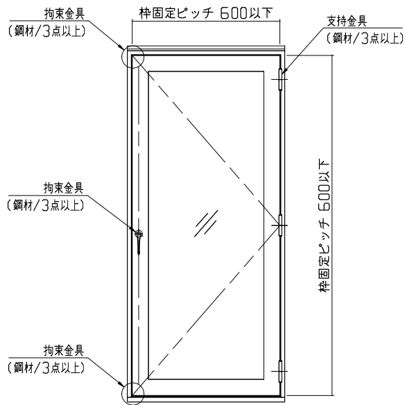
図 3-4 姿図
