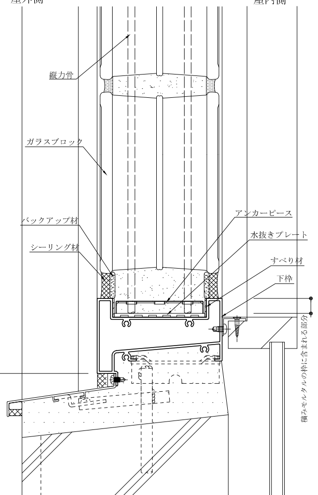
図6-⑥ 鉛直断面図
