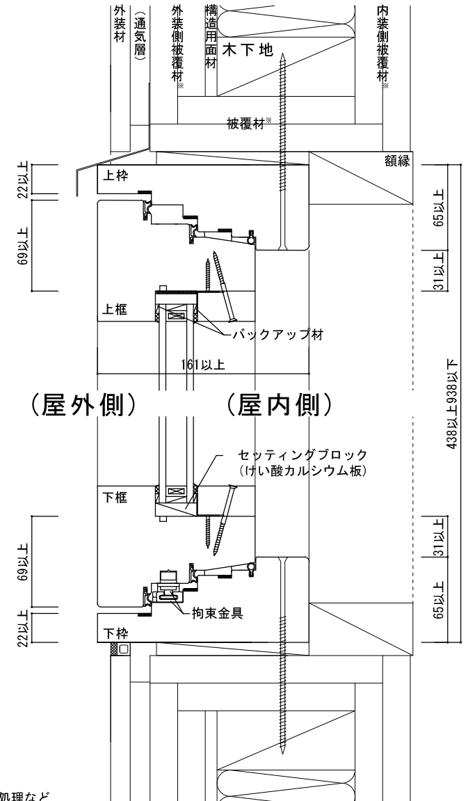
図9-④ 鉛直断面図
