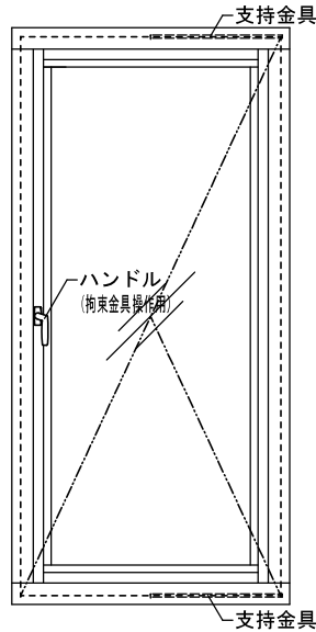
図 8 - ② 屋内側姿図
