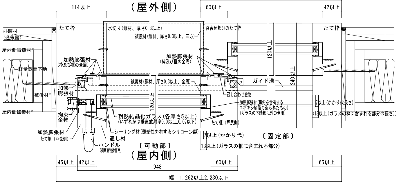
図10-⑧ 水平断面図
