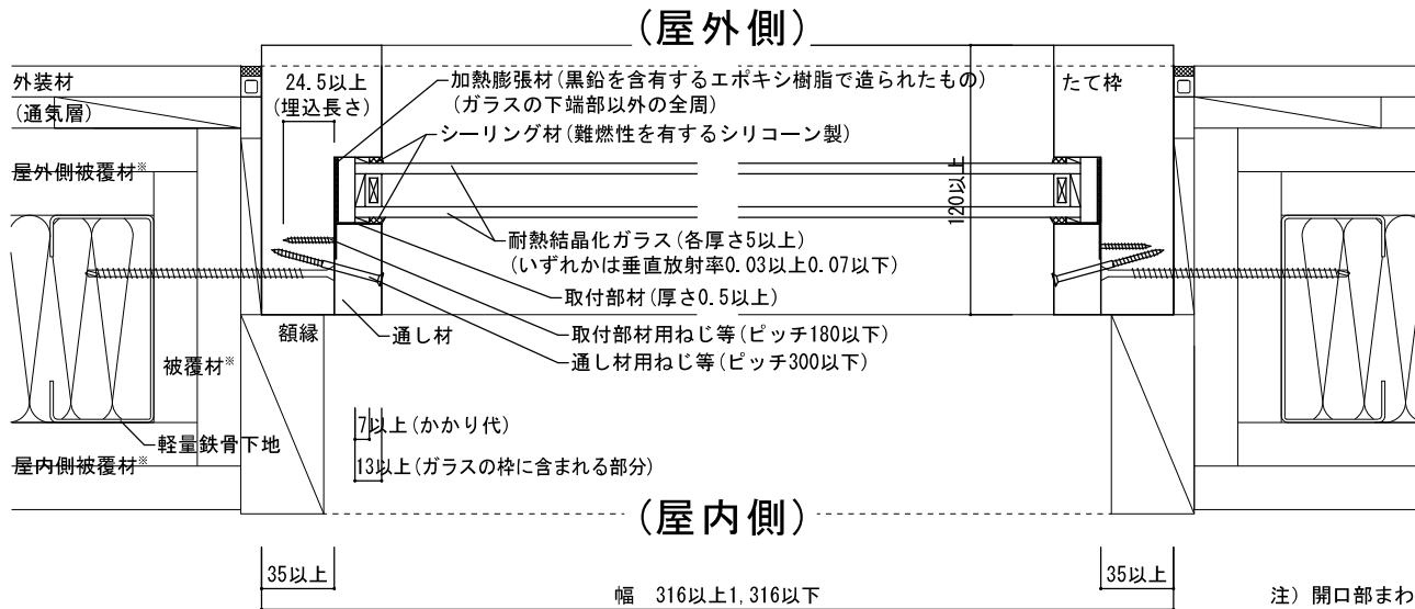
図 7-7 水平断面図
