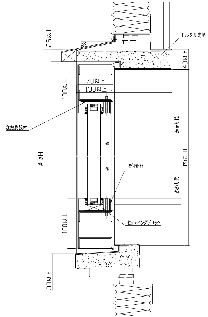
図 3-3 鉛直断面図
