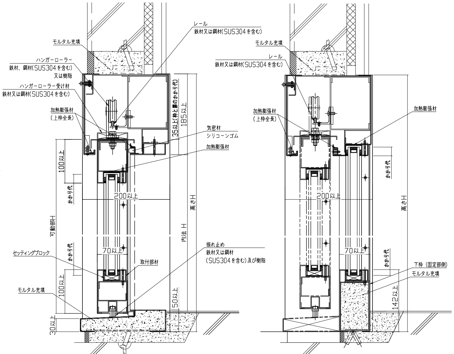
図 2-⑦ 鉛直断面図 (可動部側 (閉鎖時))
