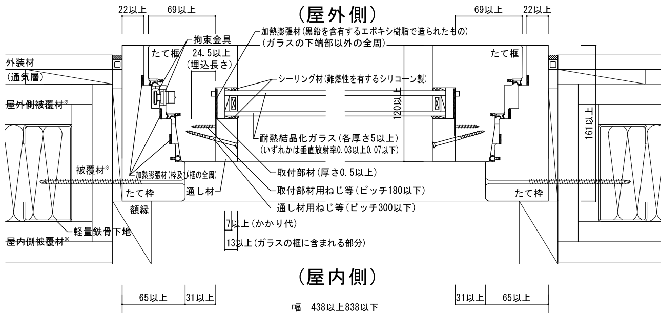
図 8 - ⑦ 水平断面図
