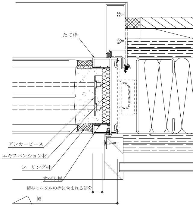
図6-② 水平断面図
