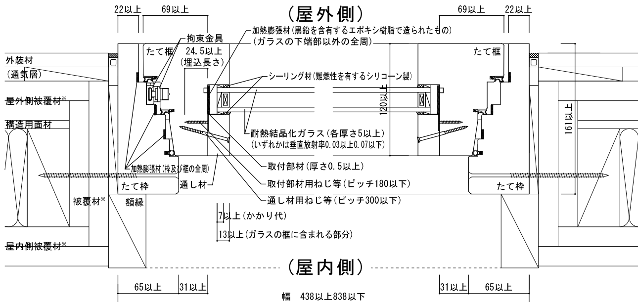
図 8 - ③ 水平断面図
