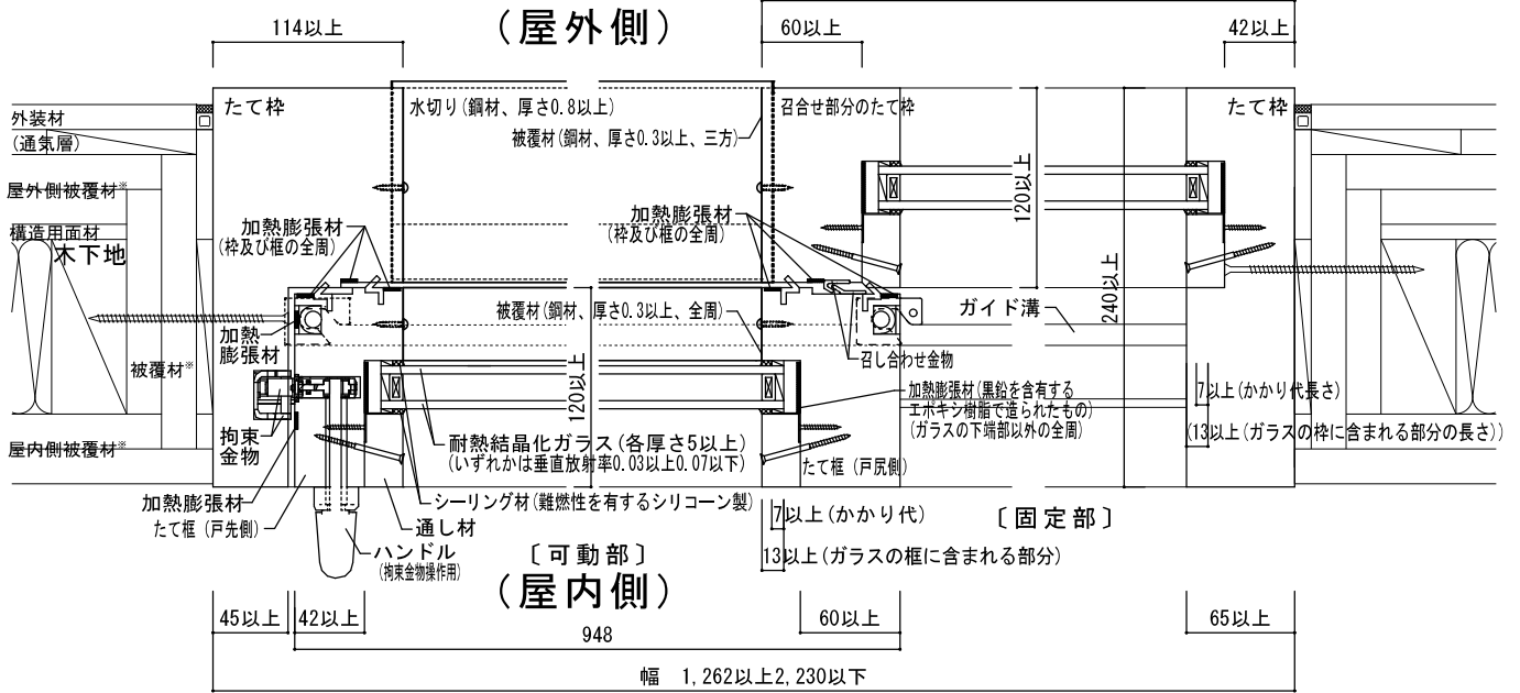
図10-⑤ 水平断面図
