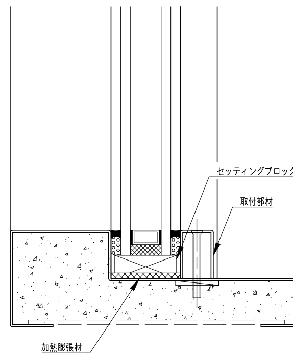
鉛直断面図
