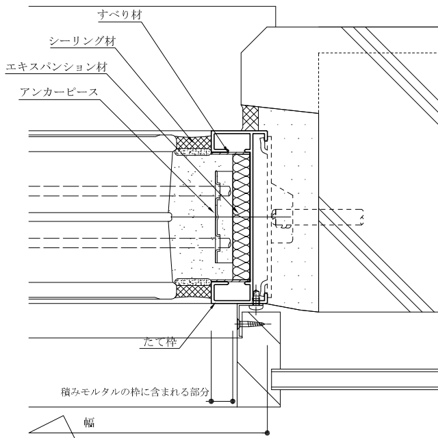
図6-⑤ 水平断面図
