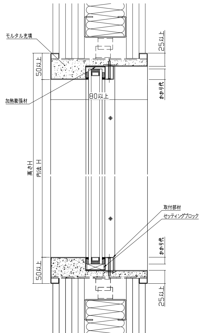
図 1-③ 鉛直断面図
