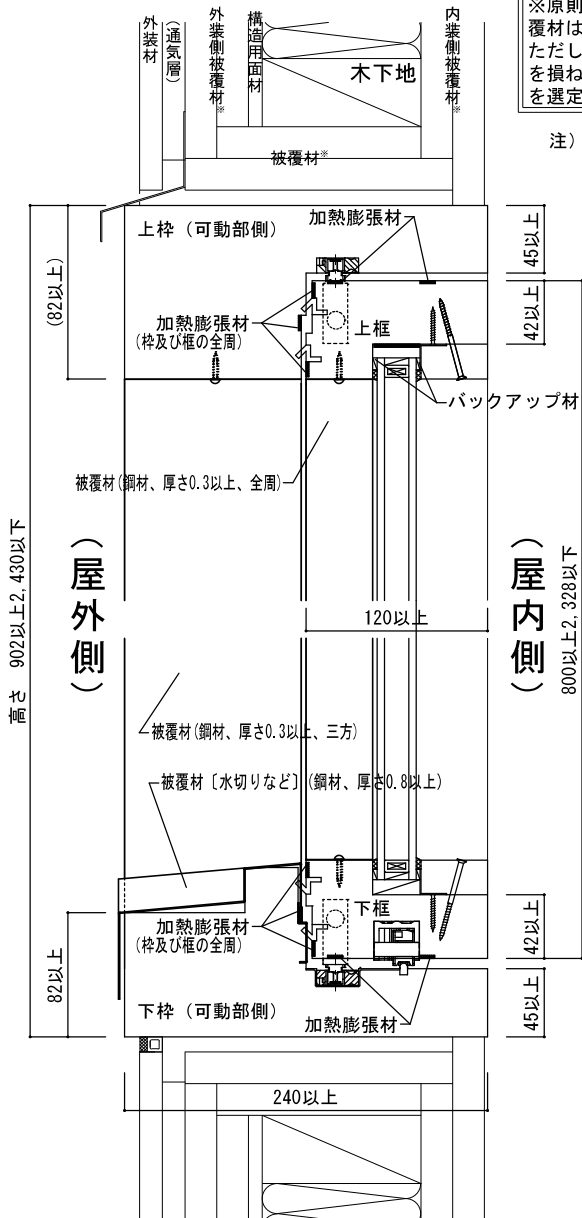
図10-⑥ 鉛直断面図〔可動部側(閉鎖時)〕
