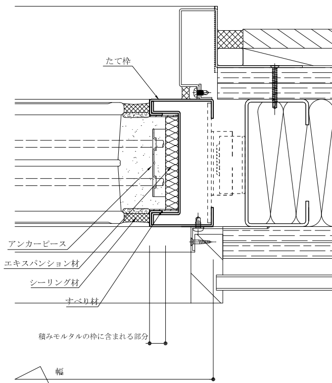
図5-② 水平断面図
